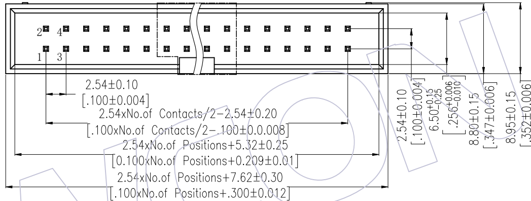
8P及以上(3个加强筋) △△
