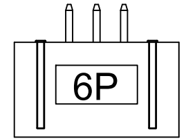
6P示意图(2个加强筋) △△
